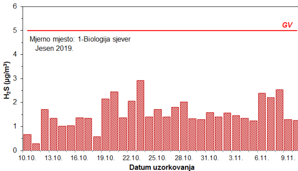
Slika 28 – Kretanje srednjih dnevnih koncentracija sumporovodika na mjernoj postaji 1 – Biologija sjever tijekom jesenskog razdoblja mjerenja
