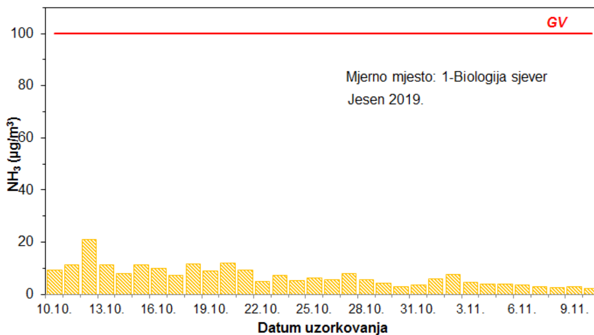
Slika 14 – Kretanje srednjih dnevnih koncentracija amonijaka na mjernoj postaji 1 – Biologija sjever tijekom jesenskog razdoblja mjerenja
