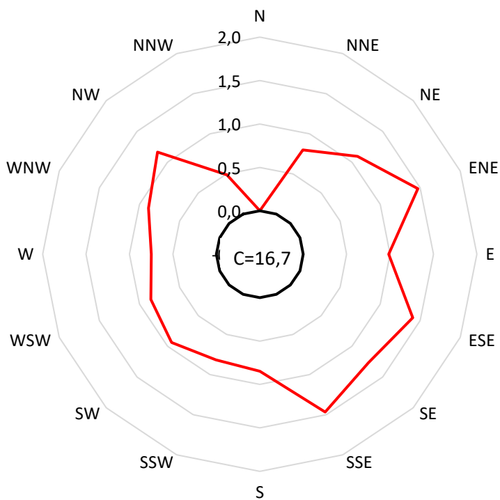
Slika 55 - Učestalost smjera vjetra [%] i srednje vrijednosti brzine vjetra [m/s] po smjerovima na mjeonoj postaji 4 – Mičevac određeni tijekom ljetnog razdoblja
