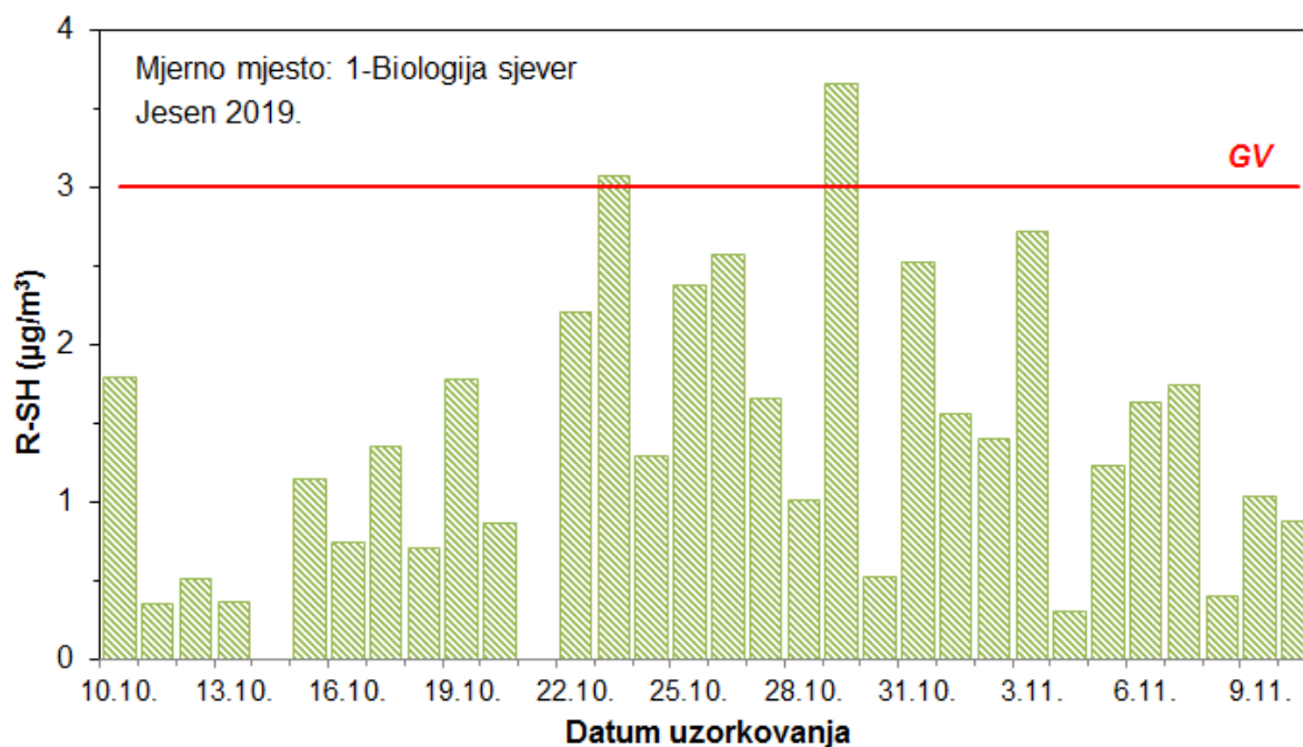
Slika 42 – Kretanje srednjih dnevnih koncentracija merkaptana na mjernoj postaji 1 – Biologija sjever tijekom jesenskog razdoblja mjerenja
