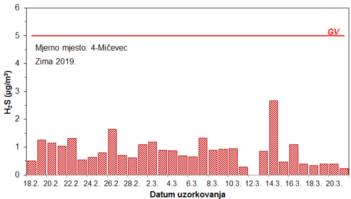
Slika 19 – Kretanje srednjih dnevnih koncentracija sumporovodika na mjernoj postaji 4 – Mičevec tijekom zimskog razdoblja mjerenja
