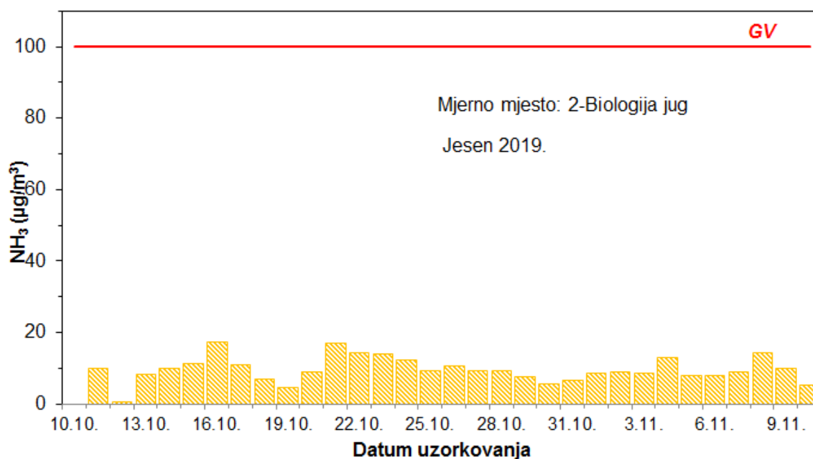
Slika 15 – Kretanje srednjih dnevnih koncentracija amonijaka na mjernoj postaji 2 – Biologija jug tijekom jesenskog razdoblja mjerenja
