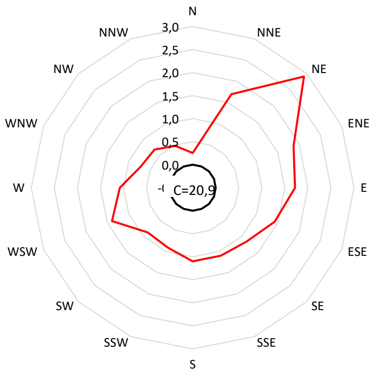
Slika 47 - Učestalost smjera vjetra [%] i srednje vrijednosti brzine vjetra [m/s] po smjerovima na mjernoj postaji 1 –Biologija sjever određeni tijekom proljetnog razdoblja
